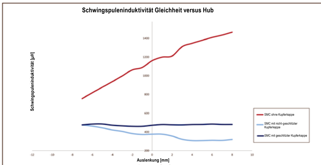
Das Diagramm zeigt die linearisierte Induktivität in der Schwingspule, die durch Schlitze in der Kupferkappe verursacht wird
