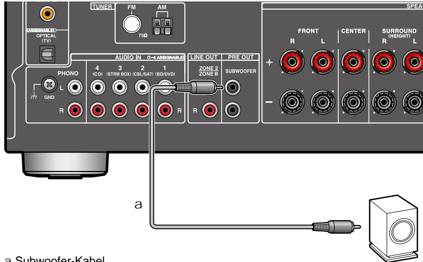
a Subwoofer-Kabel
