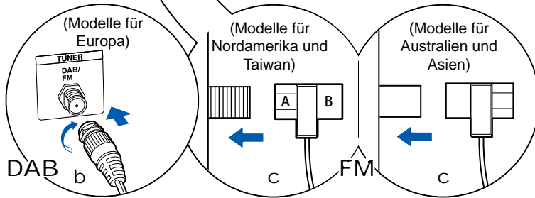
a AM-Rahmenantenne, b DAB/FM-Antenne, c FM-Zimmerantenne
