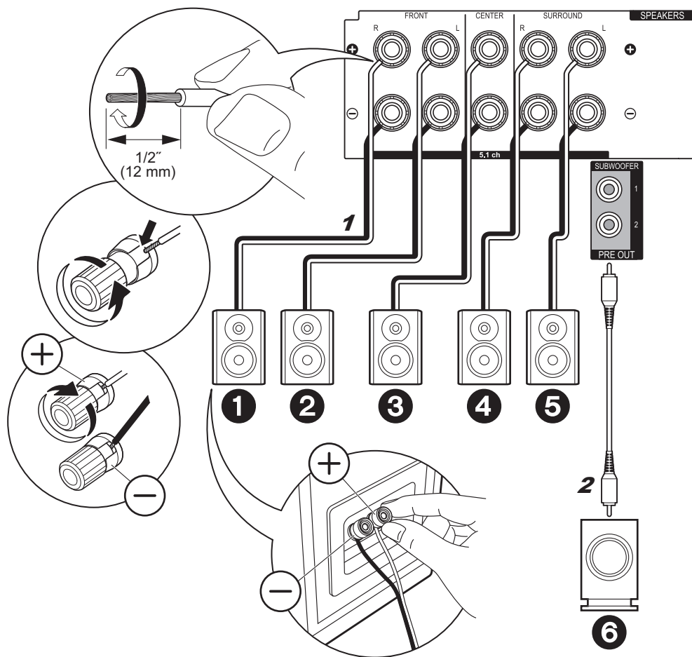
1 Lautsprecherkabel, 2 Subwoofer-Kabel
