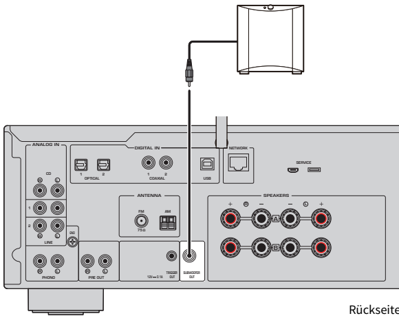
Rückseite
