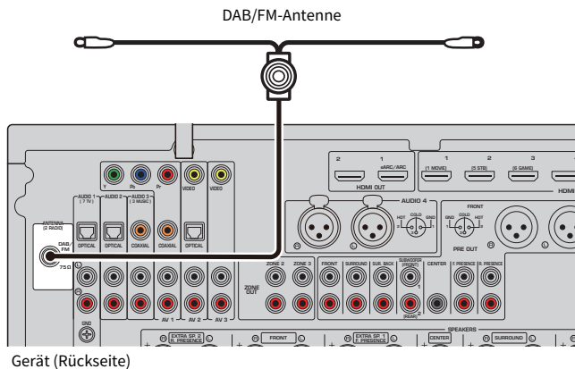
Gerät (Rückseite)
